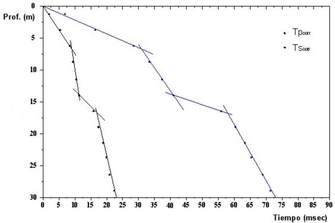
Figura 2 – Dromocrone
