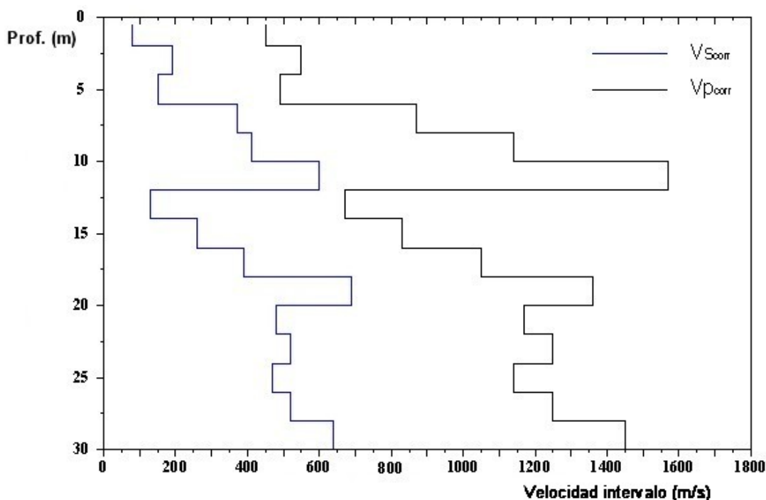
Figura 6 – Perfil de las velocidades sísmicas con el método de intervalo
