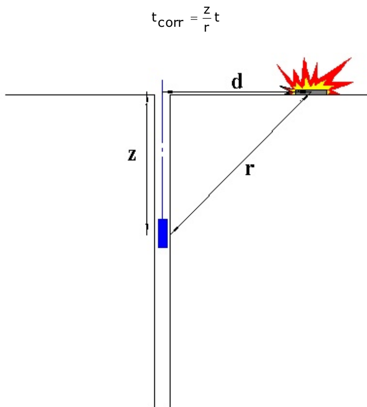
Figura 1 – Esquema de down hole con método directo
